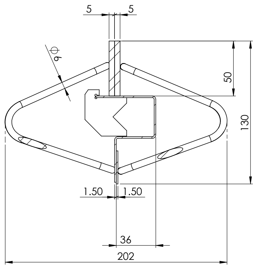
SECTION A-A SCALE 1 : 2
