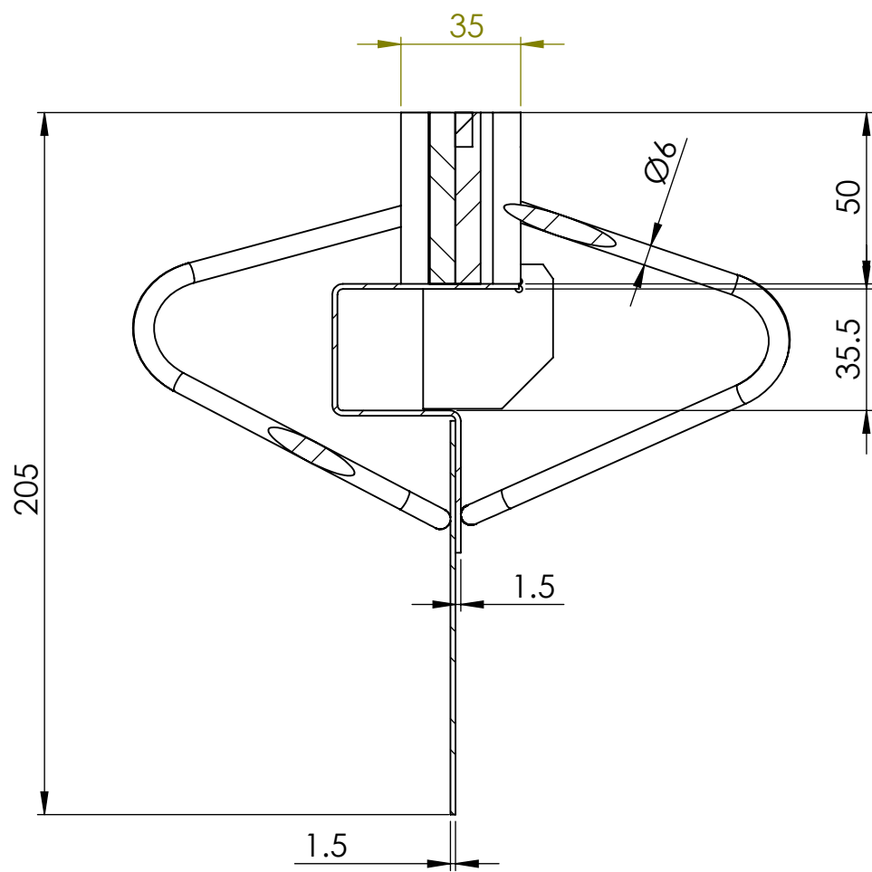
SECTION W-W SCALE 1 : 2
