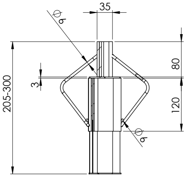
SECTION G-G SCALE 1 : 5
