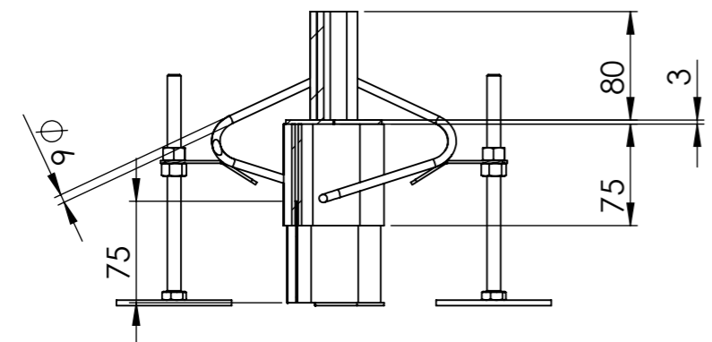
SECTION I-I SCALE 1 : 5
