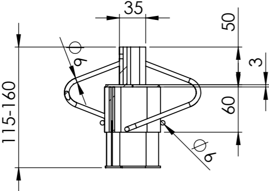
SECTION T-T SCALE 1 : 5
